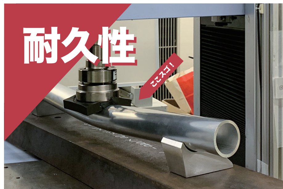
C800 フルートロング耐荷重試験
